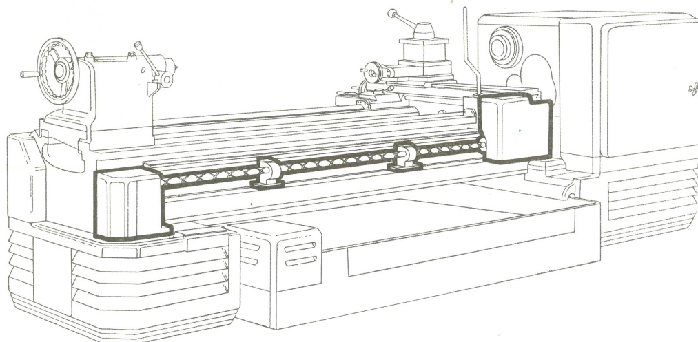
COMMANDE RAPIDE DU TRAINARD SADDLE RAPID TRAVERSE
